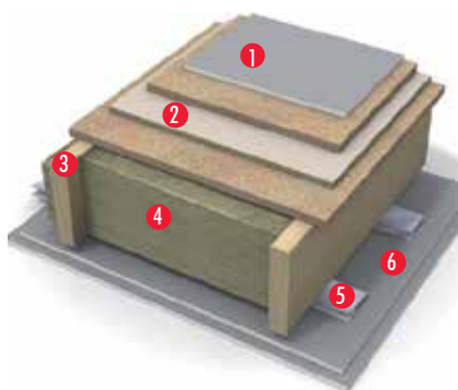
УТЕПЛЕНИЕ ДЕРЕВЯННОГО ПЕРЕКРЫТИЯ
