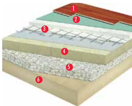
УТЕПЛЕНИЕ ПОЛА НА ГРУНТЕ
