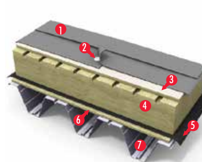
КРОВЕЛЬНАЯ СИСТЕМА PAROC AIR
