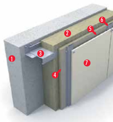
ВЕНТИЛИРУЕМЫЙ ФАСАД С ОБЛИЦОВКОЙ ИЗ ЦЕМЕНТНО- ВОЛОКНИСТЫХ ПЛИТ
