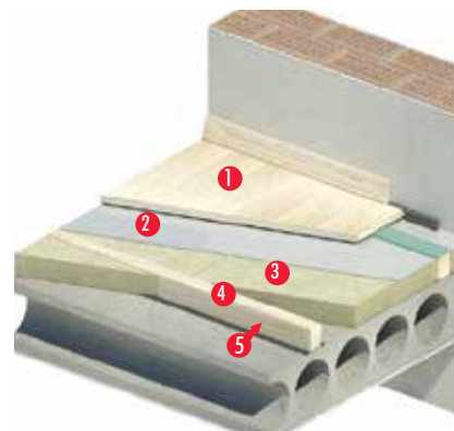
УТЕПЛЕНИЕ ПОЛА НАД НЕОТАПЛИВАЕМЫМ ПОДВАЛОМ
