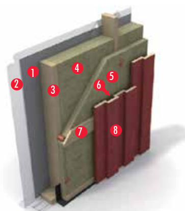
УТЕПЛЕНИЕ КАРКАСНОЙ СТЕНЫ
