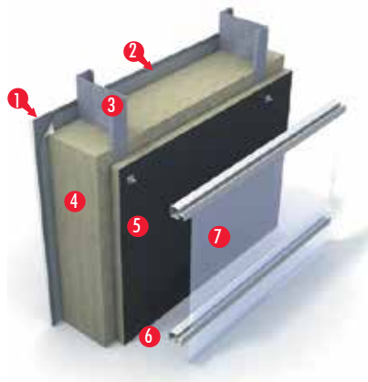
ВЕНТИЛИРУЕМЫЙ ФАСАД С ОБЛИЦОВКОЙ ИЗ СТЕКЛА
