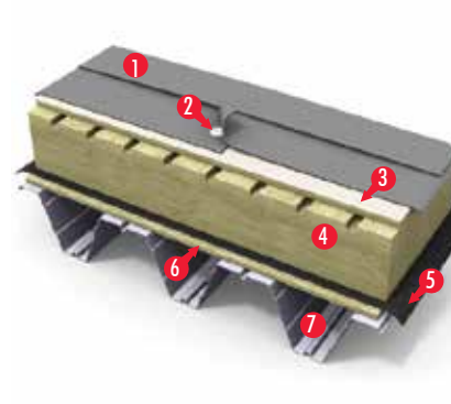
КРОВЕЛЬНАЯ СИСТЕМА PAROC AIR
