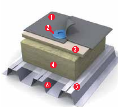
ДВУХСЛОЙНАЯ КРОВЕЛЬНАЯ СИСТЕМА
