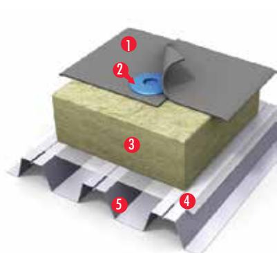
ОДНОСЛОЙНАЯ КРОВЕЛЬНАЯ СИСТЕМА
