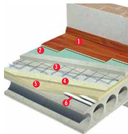
УТЕПЛЕНИЕ МЕЖЭТАЖНОГО ПЕРЕКРЫТИЯ
